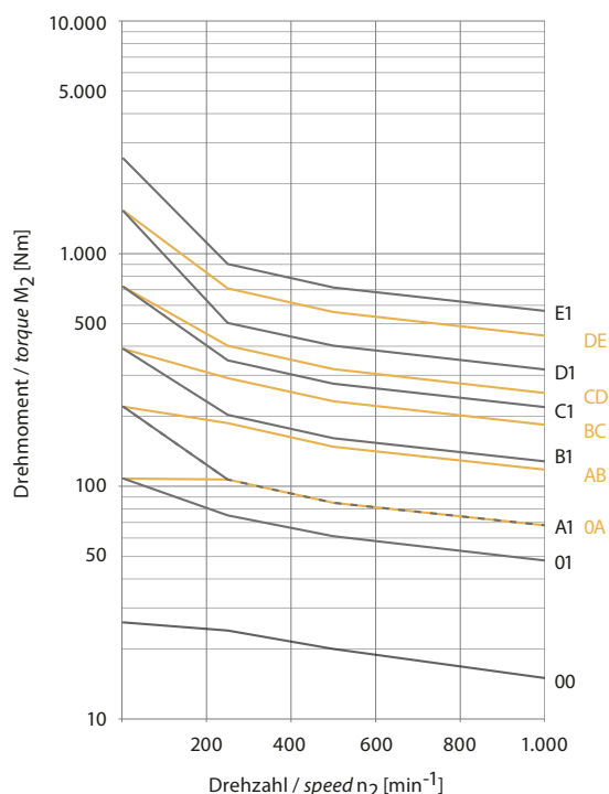
i=n_1:n_2=1:2
