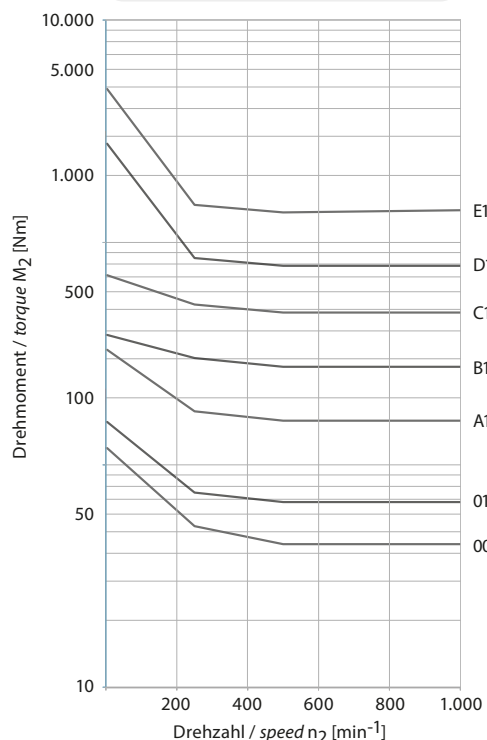
Baureihe / series PD2
