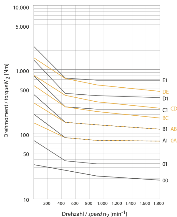
i=n_1:n_2=1:2
