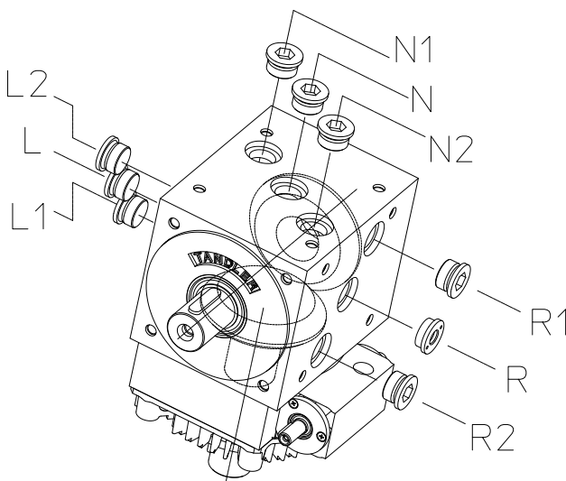
Getriebegröße / gearbox size SP2 B1 - E1
