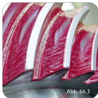
Tragbild / contact pattern Für eine optimale Kraftübertragung der Zahnflanken werden alle unsere Zahnradpaarungen anhand des Tragbildes überprüft und eingestellt. All of our gear pairs are checked and adjusted based on the contact pattern to ensure ideal power transmission from the tooth flanks.
