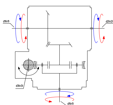
Schematische Darstellung eines SP2-Getriebes Schematic representation of an SP2 gearbox
