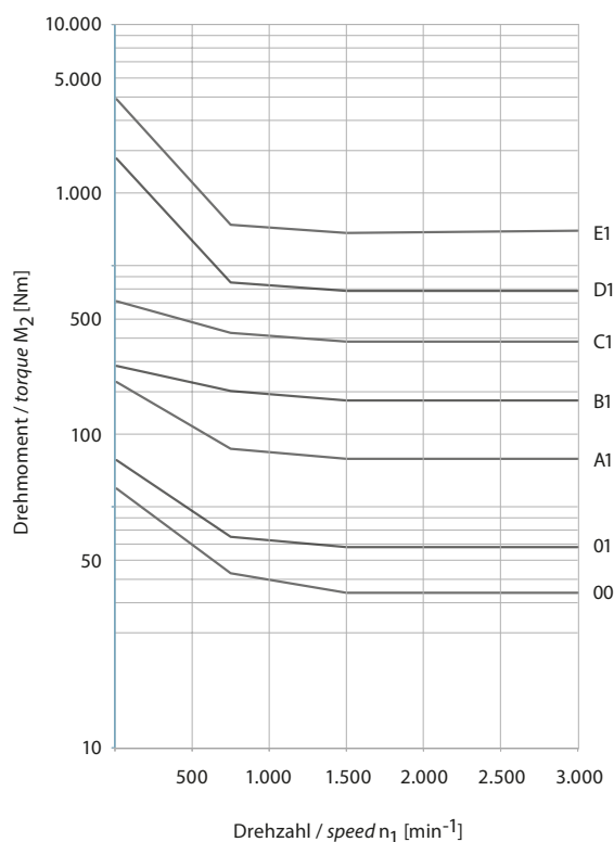
Baureihe / series PE2
