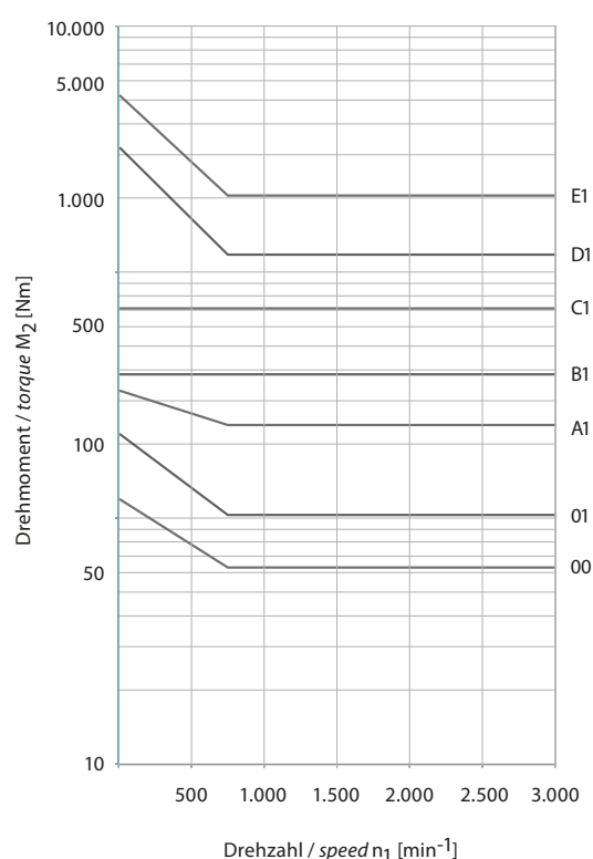
Baureihe / series PE2 - S 1508 1)
