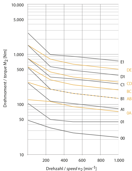
i=n_1:n_2=1:3
